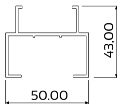
DIE No. W70223 Pivot Frame PW3
