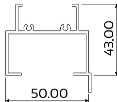
DIE No. W70222 Pivot Frame PW2
