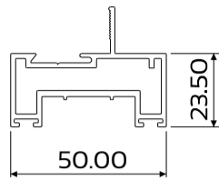
DIE No. W54787 Pivot Sash PW1
