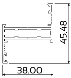
DIE No. W55717 Cas38 Tubular Sash
